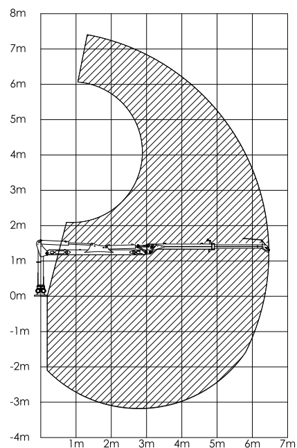
Rörelseschema
