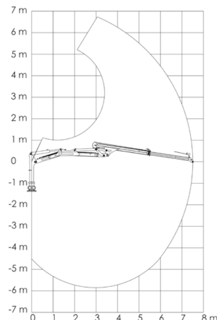
Rörelseschema
