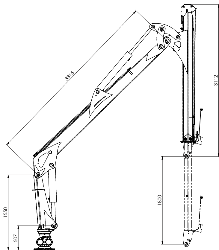
Måttskiss
