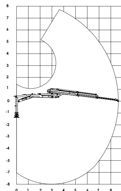
Rörelseschema
