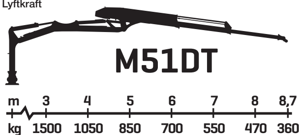
Lyftkraft
